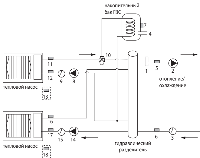
Пример 3. Система отопления и охлаждения с использованием гидромодулей Escodan
