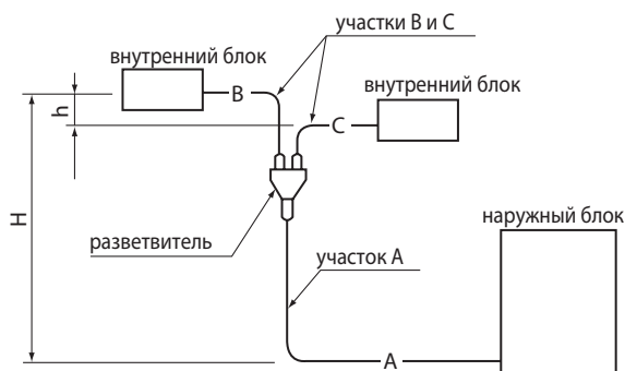
Система 1:2
